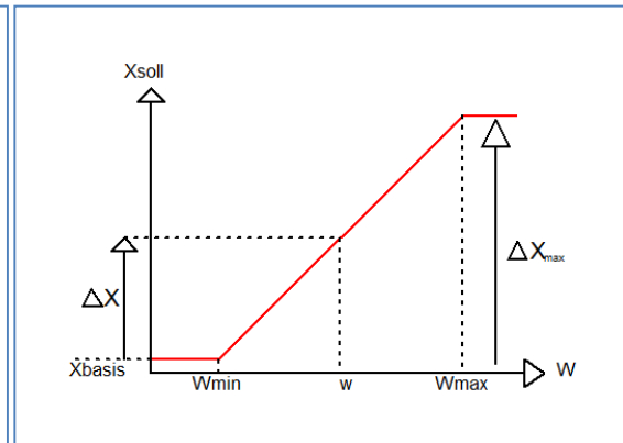
Abbildung 21: Beispiel – Führung Anhebung
