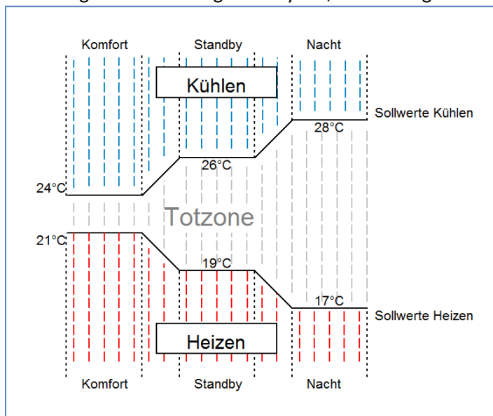
Abbildung 16: Beispiel Totzone und resultierende Sollwerte
