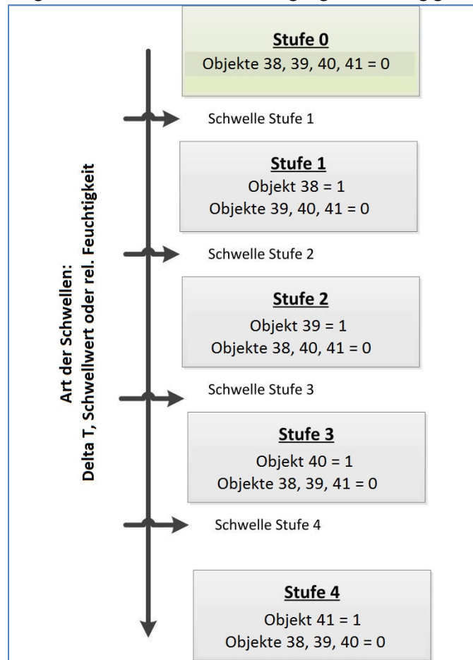
Abbildung 34: Schaltverhalten – Stufenschalter
