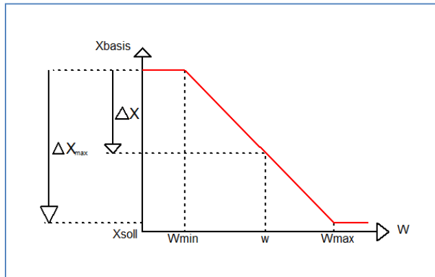
Abbildung 20: Beispiel – Führung Absenkung
