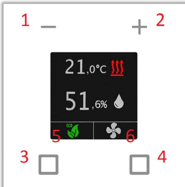
Abbildung 42: Beschreibung Tasten/Anzeige
