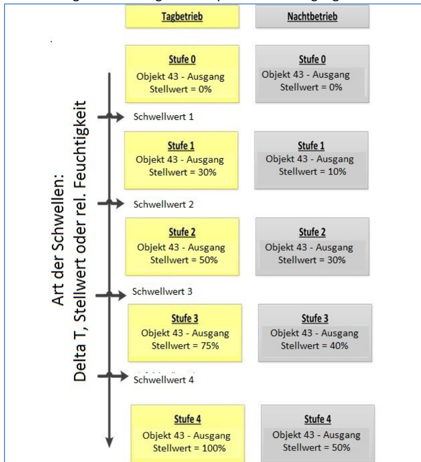
Abbildung 40: Beispiel Ausgang – Stufenschalter als Byte
